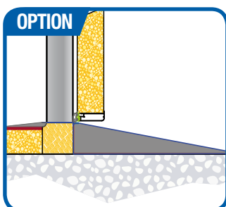
Con rampa interna ed esterna - With internal and external ramp - Avec rampe intérieure et extérieure - Mit innerer und äußerer Rampe
